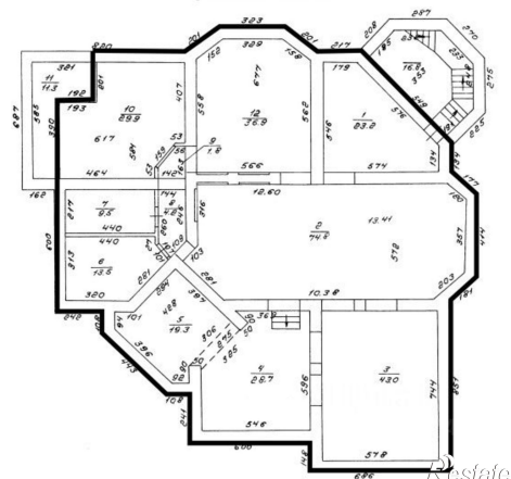
Подвал Н - 3.30
