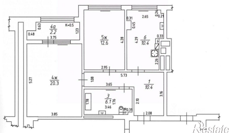
7-ЭТАЖ H=2.60
