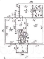
ПОДВАЛ Н- 1,70
