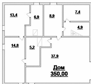
Подвал Н=2,50
