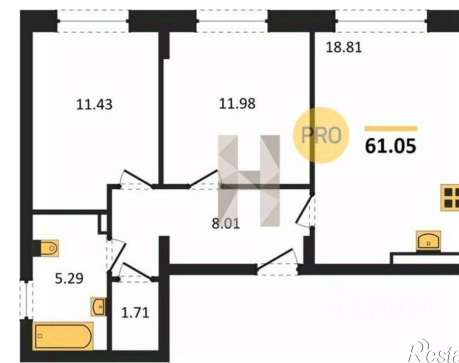
КОРПУС 1 Секция 4 План 7-9 этажей
